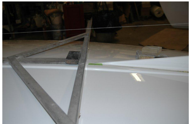
Figures H.1.4.1 & H.1.4.2 String Baseline
